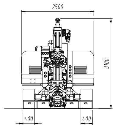
Peso totale unità /Machine total weight / Gesamtgewicht der Einheit/Poids total de l'unité ~ 14000 kg (30800 lbs)
